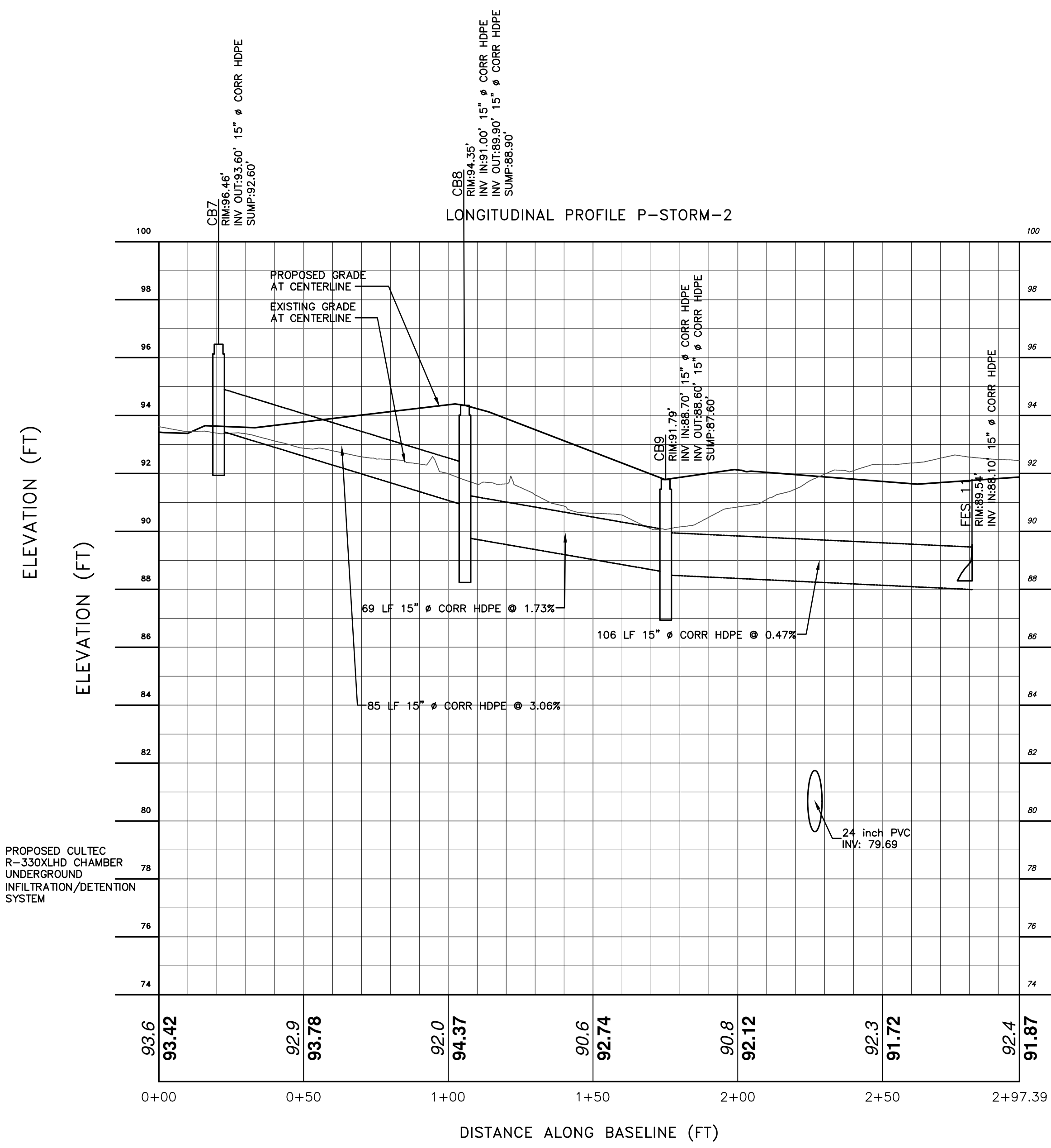
STORM LINE 2 PROFILE SCALE: 1" = 3'V 1" = 30'H
