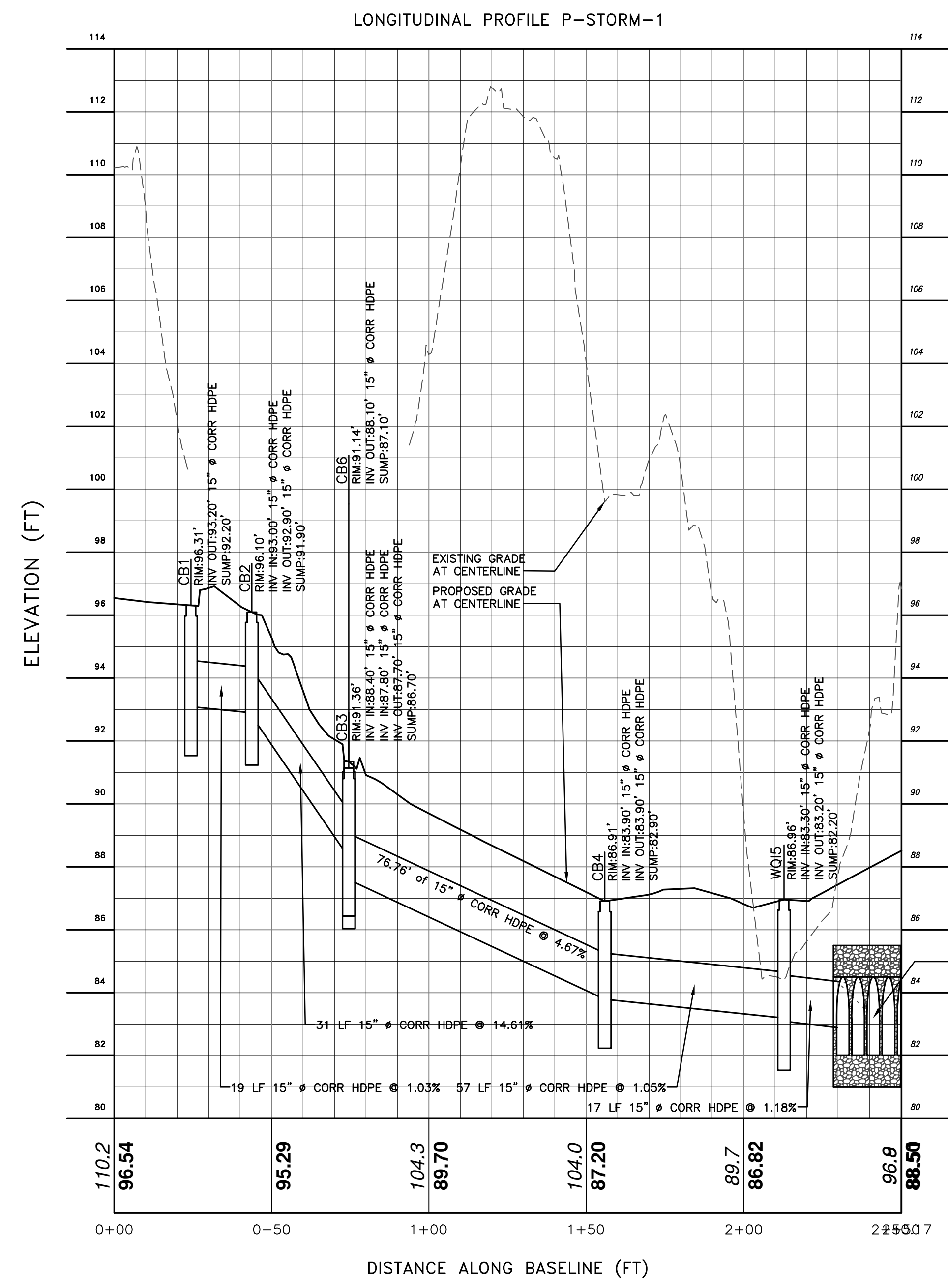
STORM LINE 1 PROFILE SCALE: 1" = 3'V 1" = 30'H
