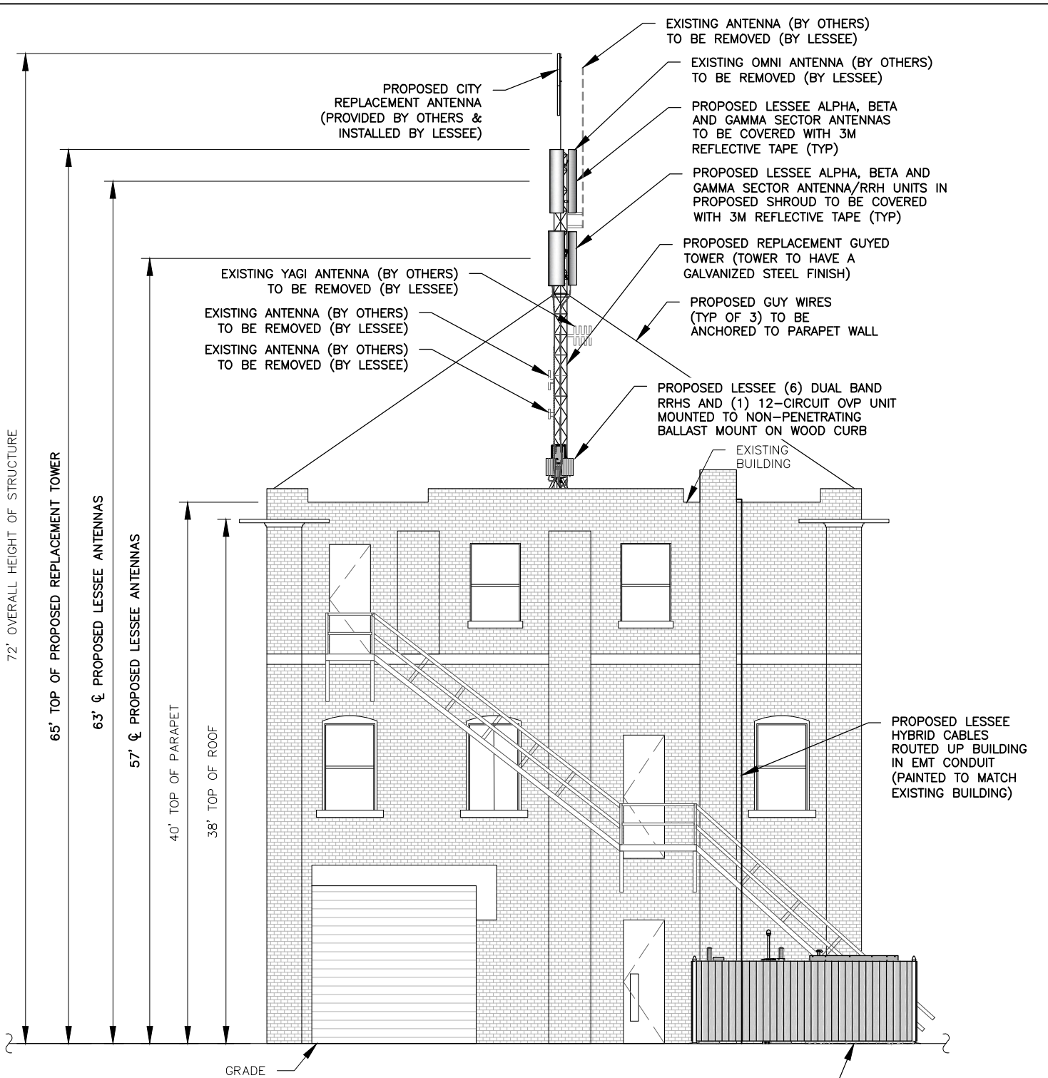
1 ELEVATION LE-4 SCALE: 1" = 10'
