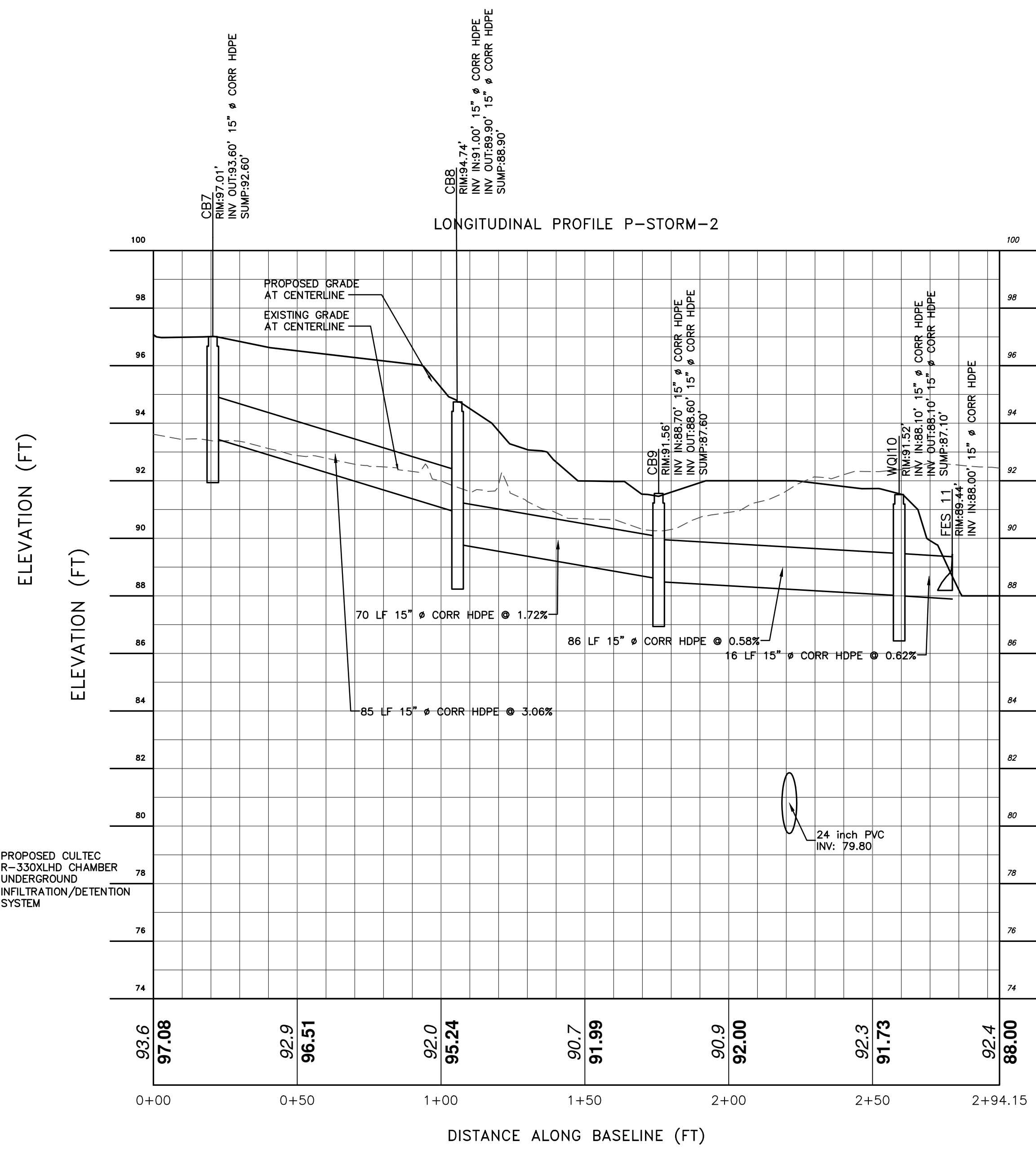
STORM LINE 2 PROFILE SCALE: 1" = 3'V 1" = 30'H
